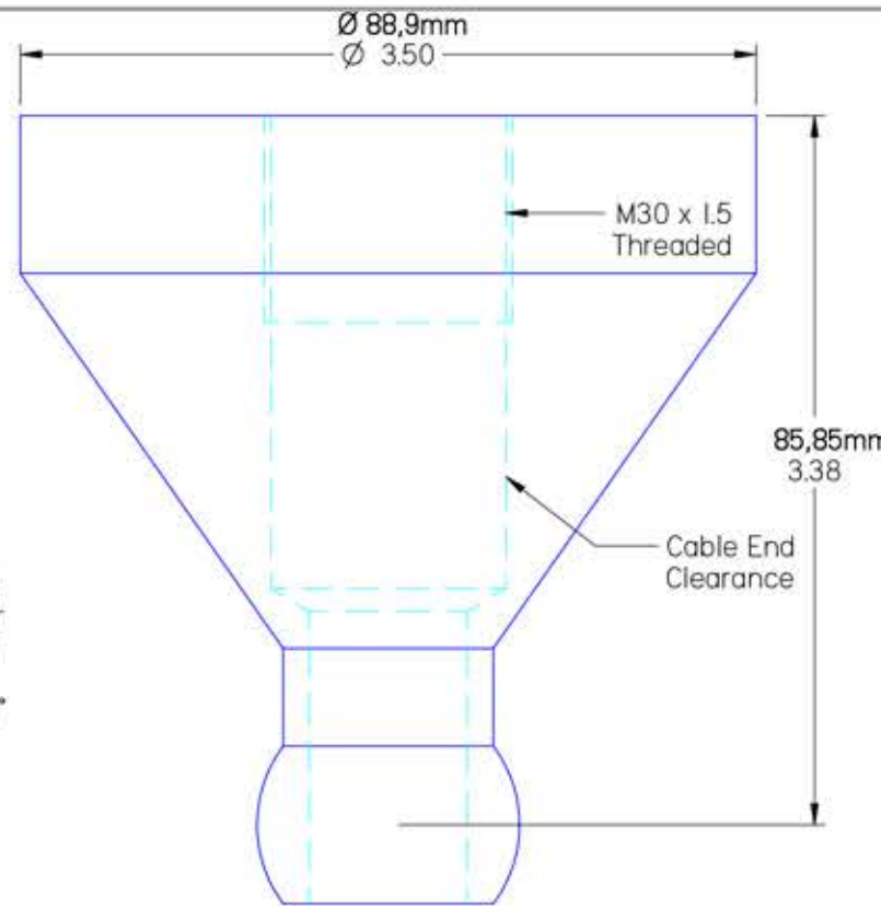
AFSB-4 Button Base
